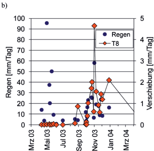
Fig. 3: a) Abhängigkeit der Verschiebungen oberflächlich versetzter Jointmeter T vom Niederschlag (Regressionsgeraden); b) In der kalten Jahreszeit, wo in den infolge des Temperaturrückgangs am stärksten geöffneten Klüften ein kritischer Kluftwasserdruck aufgebaut werden kann, vermögen Niederschläge Verschiebungsschübe auszulösen. Gleiche und höhere Niederschlagsmengen bleiben im Sommer dagegen wirkungslos (Daten von Niederschlagsperioden mit \pm unveränderter, mittlerer 24 h-Temperatur, Val d'Infern [2]).
