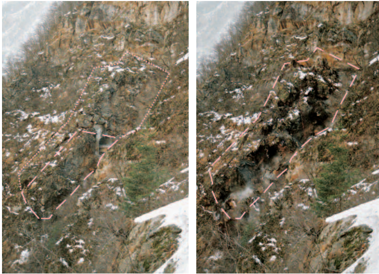
Fig. 5b: Im «Kipp/Gleit»-Prozess erfolgt das Versagen als erstes in der Kriech- oder Bruchzone in dem im Feld meist kaum lokalisierbaren Fuss der Sturzmasse. Die in der Folge hängende Ablösezone folgt dem Sturzereignis hinterher (Val d'Infern [6]).
