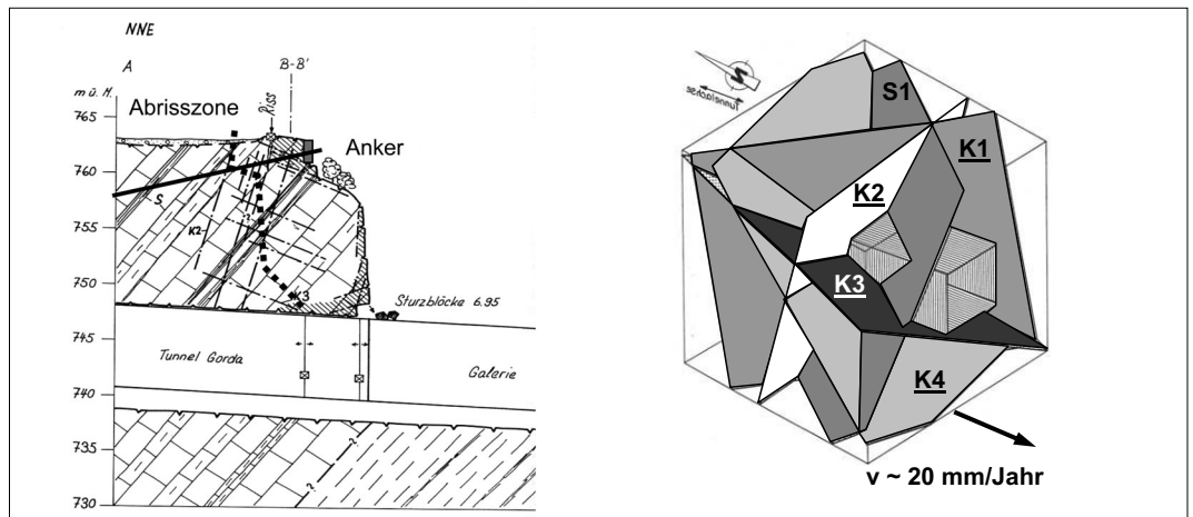
Fig. 15: Schnitt durch die Tunnelachse mit der Abrisszone. Die Felstrennflächen im Blockdiagramm zeigen die Felsablösung entlang der K2/K1 Klüfte und der Gleitfläche K4 mit 50° Neigung Richtung Süd.
