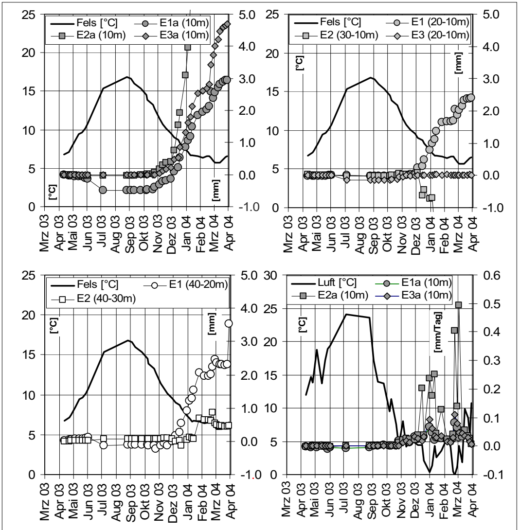
Fig. 10: Die Extensometer zeigen nur bis in Felstiefen von ~10 m temperaturabhängige Verschiebungen (Oben, unten links). Da das Extensometer E1 vom Tunnelinneren Richtung Felsoberfläche versetzt wurde, zeigt es auch in den längeren Teilstrecken Deformationen. Bei mittleren Tageslufttemperaturen unter 5°C erfolgt eine starke Zunahme der Verschiebungsraten (unten rechts).
