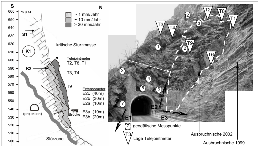
Fig. 5: Dank der Messanlage konnte in der Felsrippe eine kritische Sturzmasse von \sim 3'000 \text{ m}^3 und in die Felstiefe Entfestigungszone mit abnehmenden Verschiebungsraten erkannt werden.
